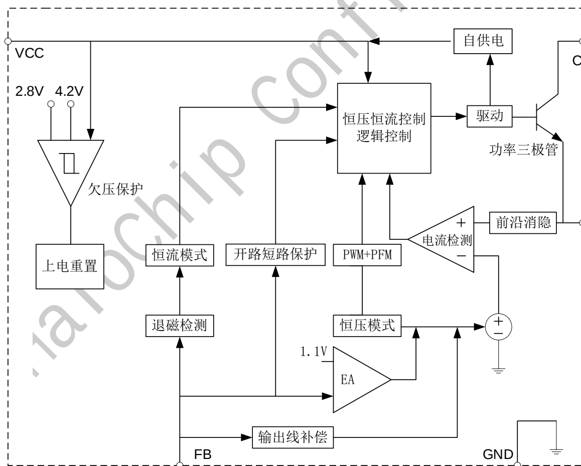
图 3 GP8891CAS 内部框图
