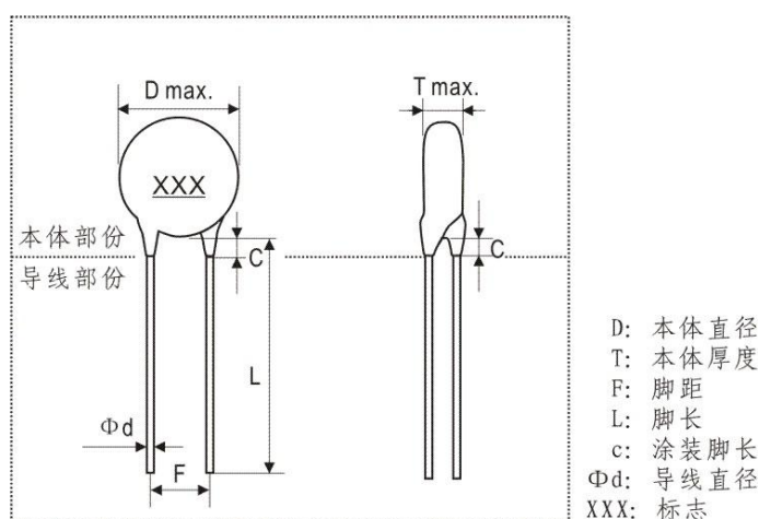
安规陶瓷电容器结构图
