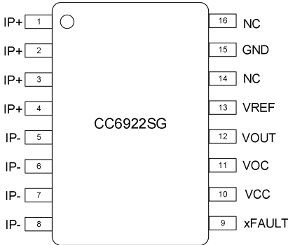
SOP16W 封装
