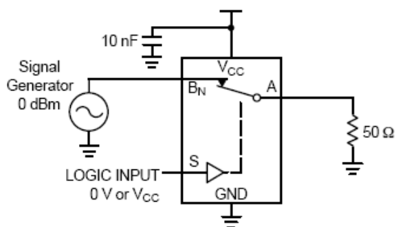
图 8 带宽
