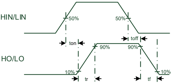
图 5-1 时序参数 t_{on}/t_{off}/t_r/t_f 定义
