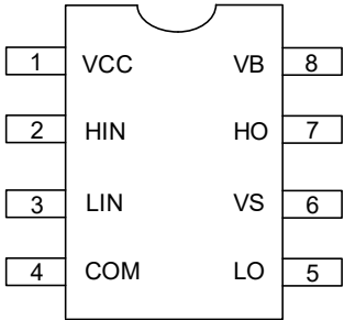
图 2-1 LKS571 管脚分布图
