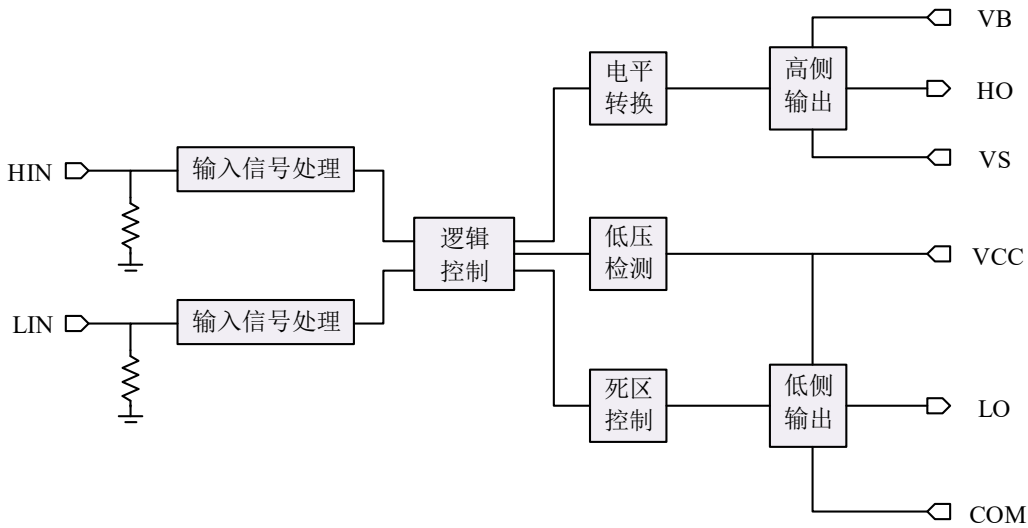
图 1-1 LKS571 内部结构框图
