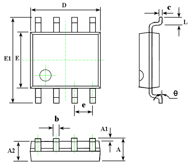
图 3-1 LKS571 封装图示
