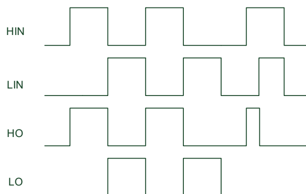
图 1-2 LKS571 控制逻辑时序图
