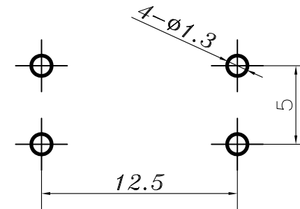
PCB. 焊接图
