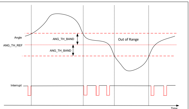
图 7-9. MAG_THR_DIR = 1b 、 THR_SEL=01b 、 INT_STATE=1b 时的角度限值交叉检查
