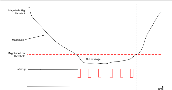
图 7-7. MAG_THR_DIR = 1h 、 THR_SEL[1:0] = 3h 、 INT_STATE = 1h 时的磁体限值交叉检查
