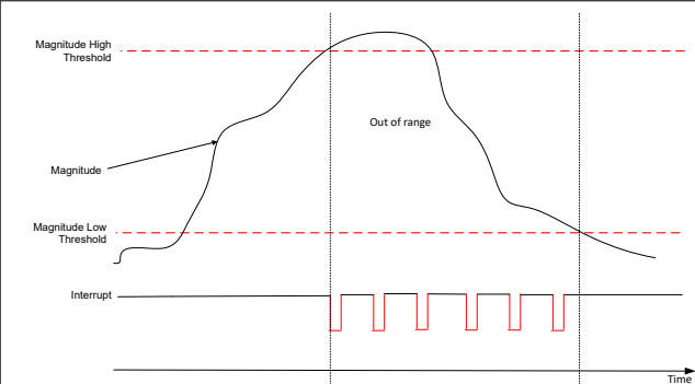
图 7-6. MAG_THR_DIR = 0h 、 THR_SEL[1:0] = 3h 、 INT_STATE = 1h 时的磁体限值交叉检查
