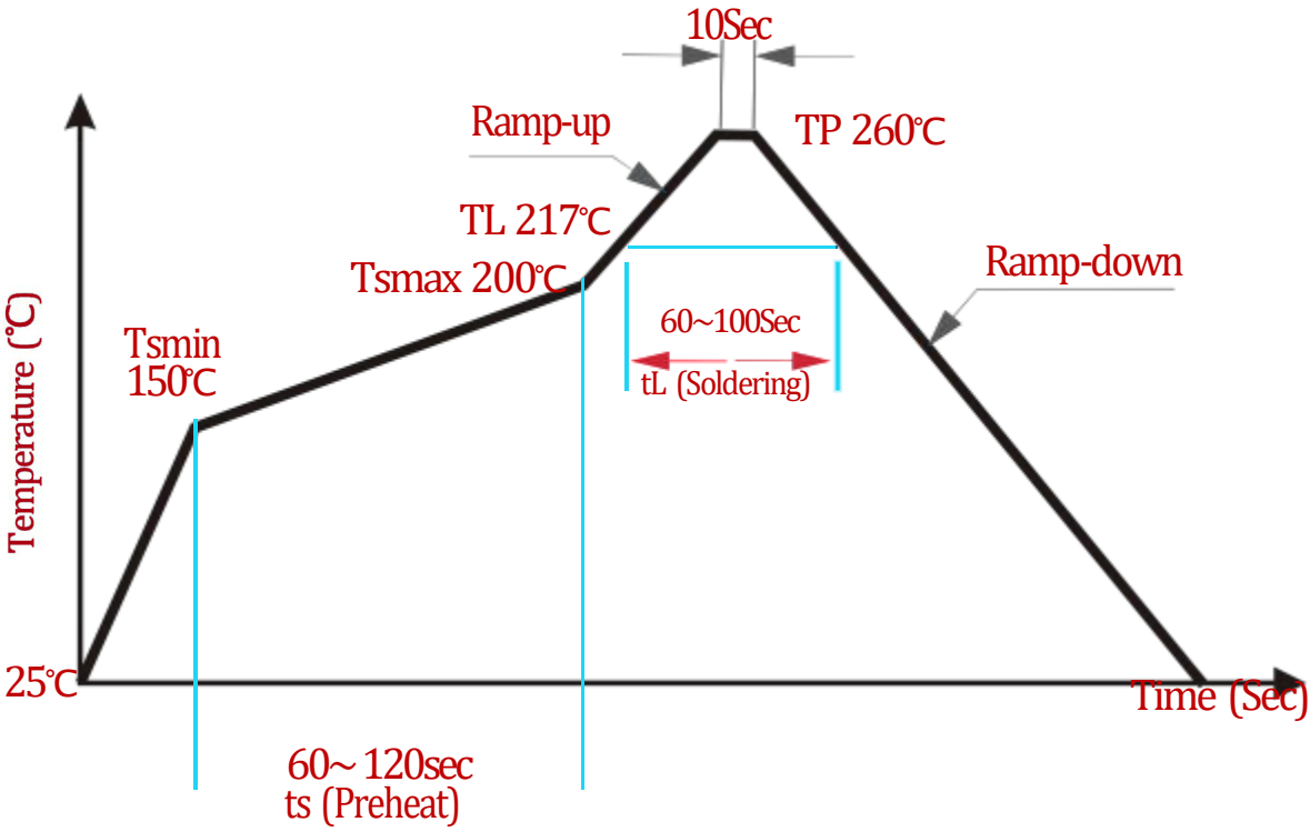
回流焊曲线
