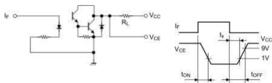
Fig. 1开关时间测试电路
