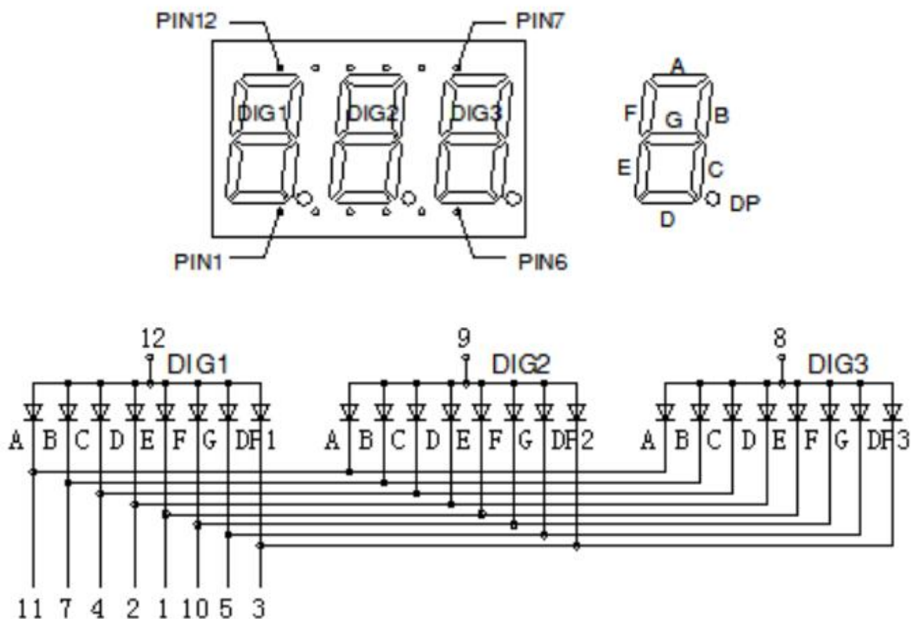
D3631A/B原理图
