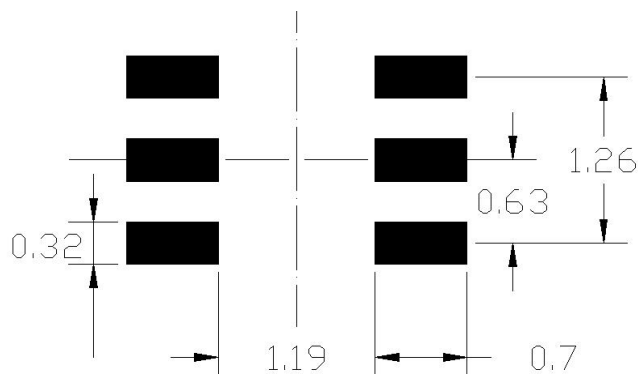
建议焊盘尺寸(单位: mm)
