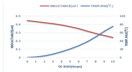
AFE201612SR47MBT
