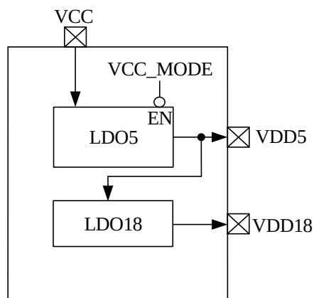
图 29-1 电源模块功能框图
