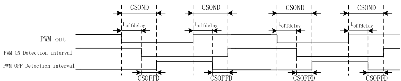
图 14-5 采样区间图
