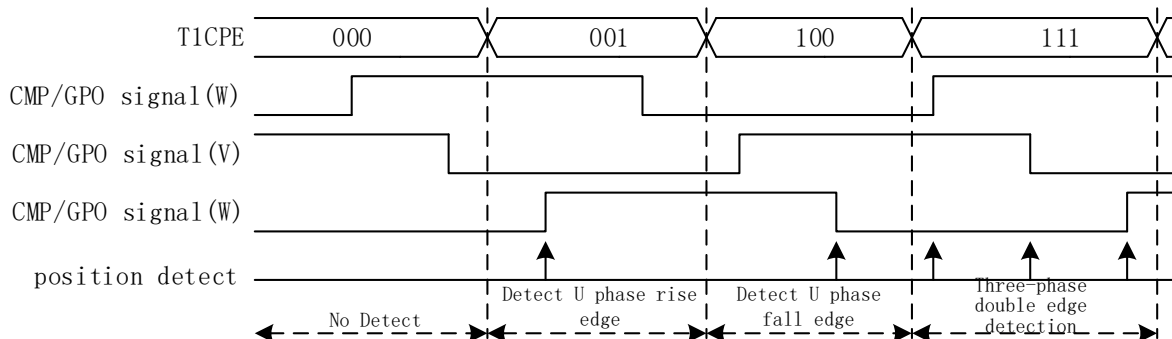
图 14-6 位置检测时序图
