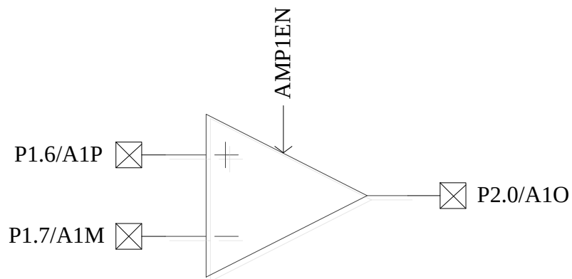
图 27-4 AMP1 输入输出相关端口
