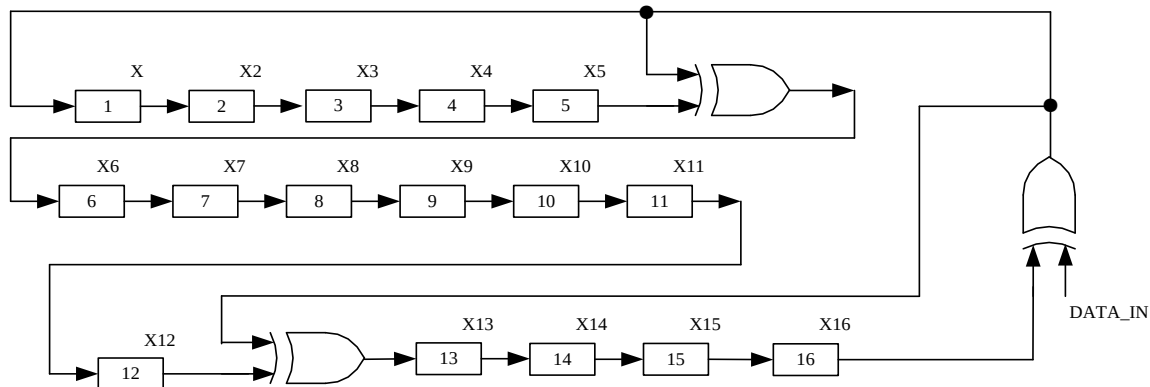
图 31-2 CRC16 电路原理图
