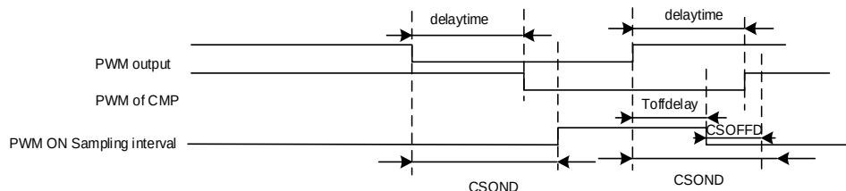
图 28-14 PWM OFF 采样模式
