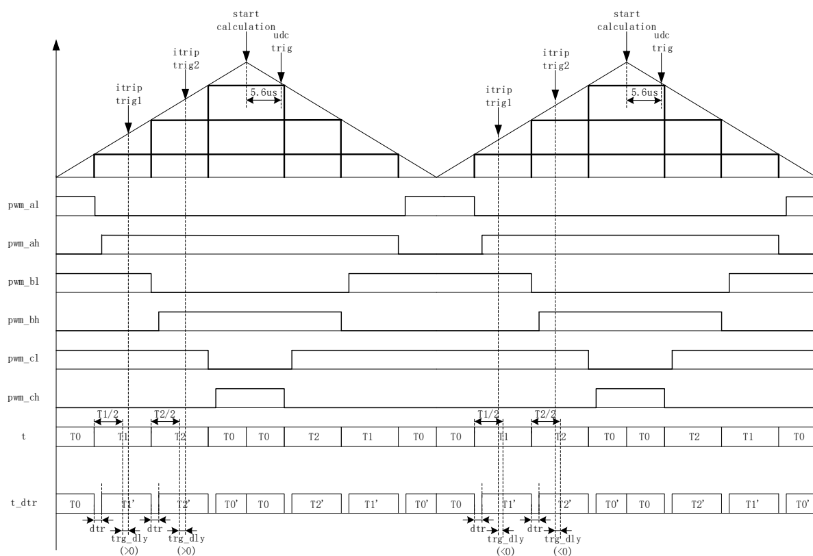
图 13-10 单电阻采样时序
