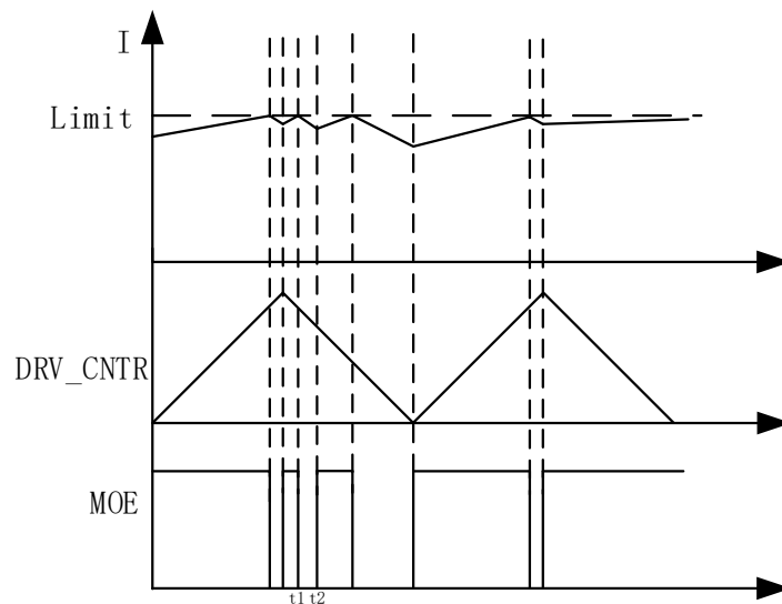
图 28-6 EVT_FILT[MOEMD] = 11，逐波限流波形( t_2 - t_1 = 5\mu\text{s} )
