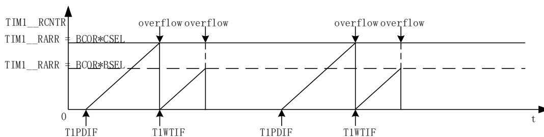
图 14-4 重载计数器计数波形图
