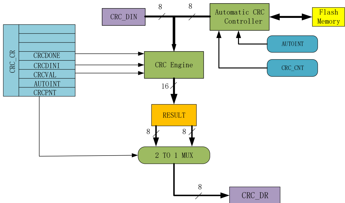
图 31-1 CRC 功能框图
