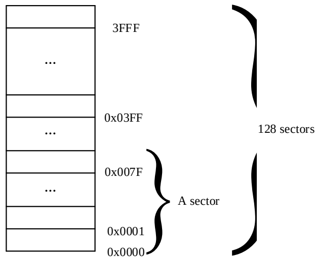
图 31-3 ROM 访问分区图
