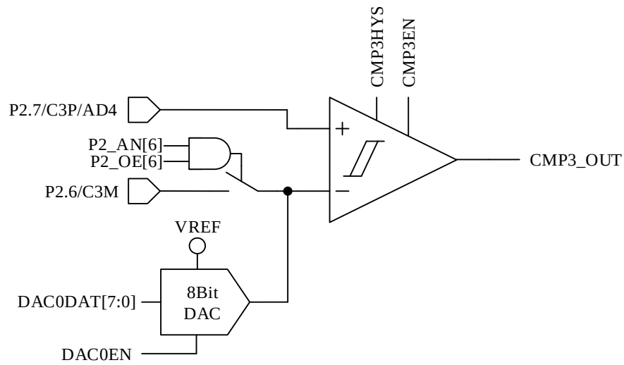
图 28-2 单比较器输入模式
