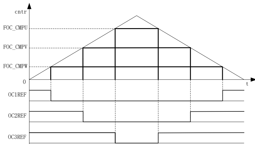
图 18-3 PWM 生成图
