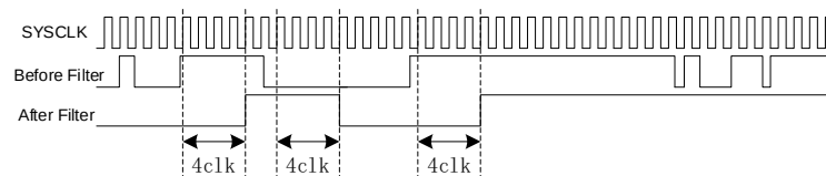
图 15-4 滤波模块时序图
