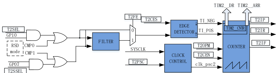
图 15-5 输入 timer 模式原理框图
