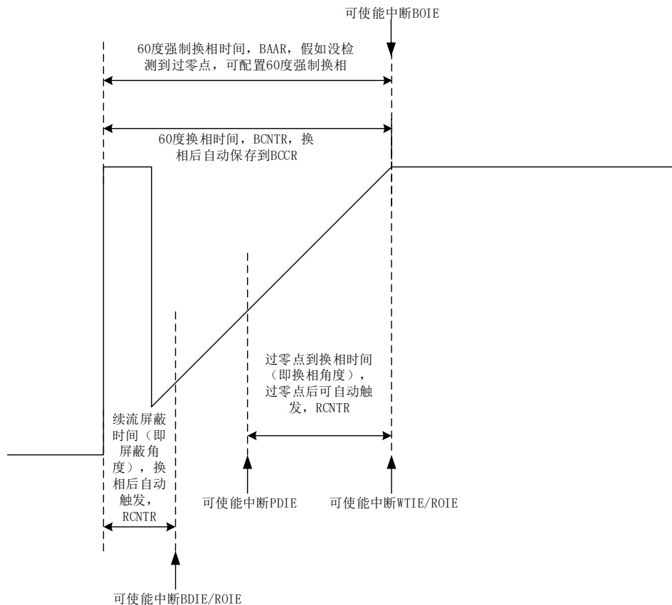
图 14-6 BLDC 的工作原理
