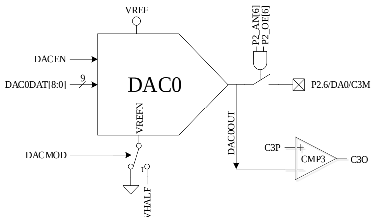
图 23-1 DAC0 功能框图
