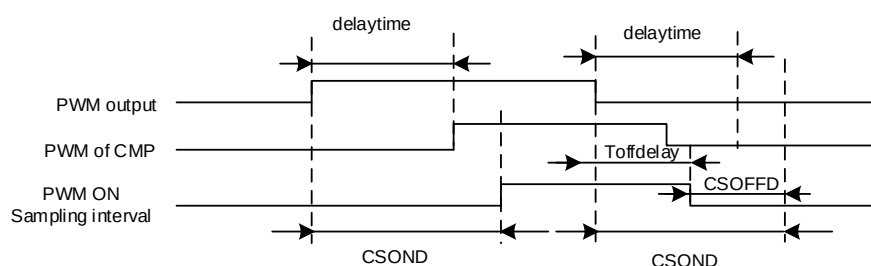
图 15-11 PWM ON 采样模式
