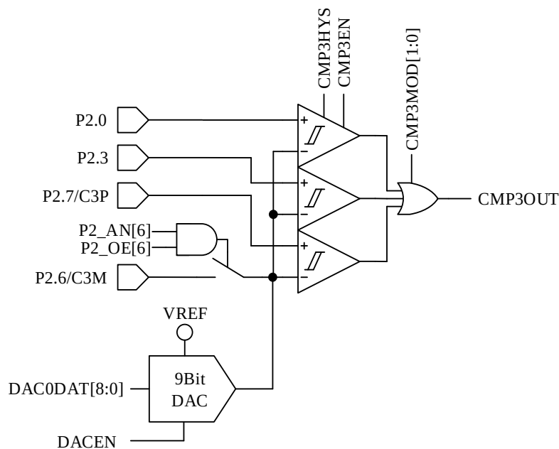
图 28-4 三比较器输入模式
