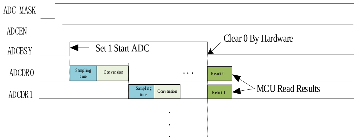
图 22-3 ADC 顺序采样时序图
