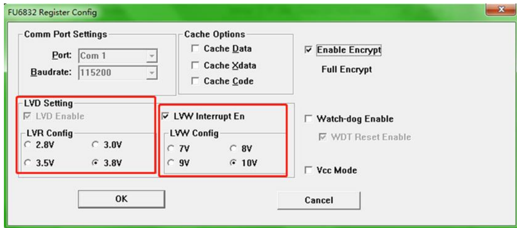
图 29-4 低电压预警电压、中断配置以及低电压复位电压设置
