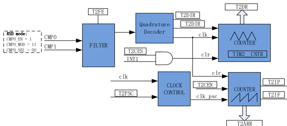
图 15-9 RSD 模式原理框图
