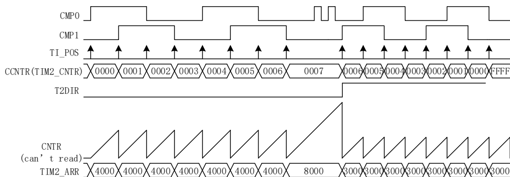
图 15-10 RSD 模式时序图
