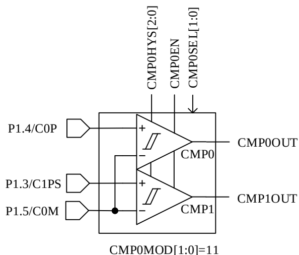
图 28-12 双比较器模式
