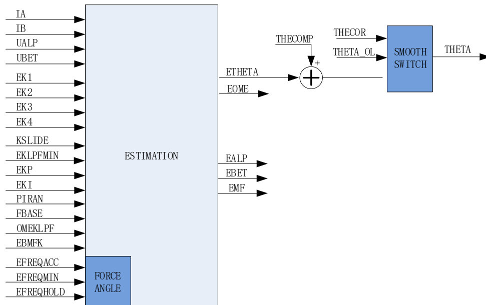
图 13-14 估算器原理框图
