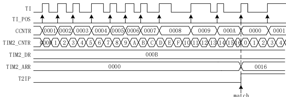
图 15-8 输入计数模式时序图
