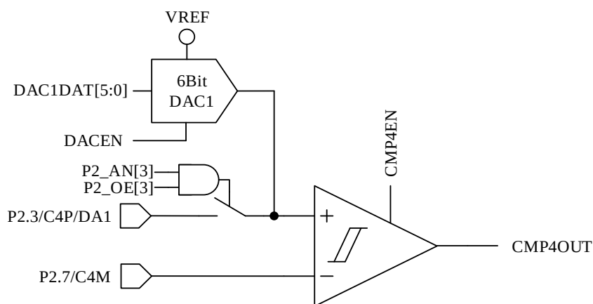
图 28-7 CMP4 模块示意图
