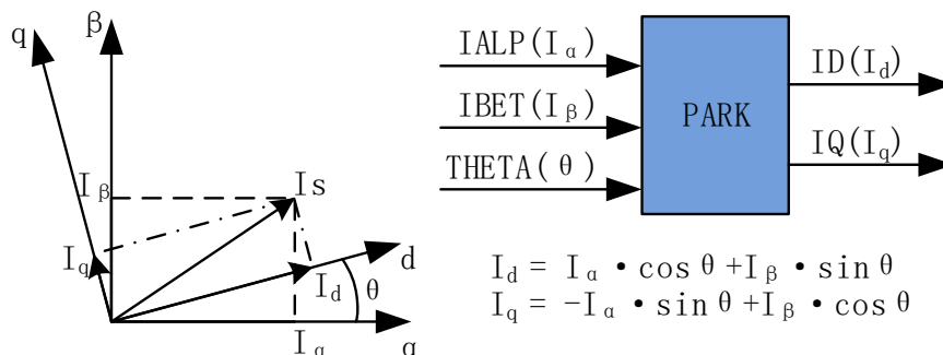
图 13-5 Park 变换
