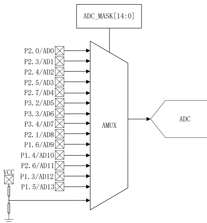
图 22-1 ADC 多路复用器框图
