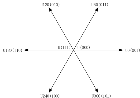
图 13-6 SVPWM 电压矢量
