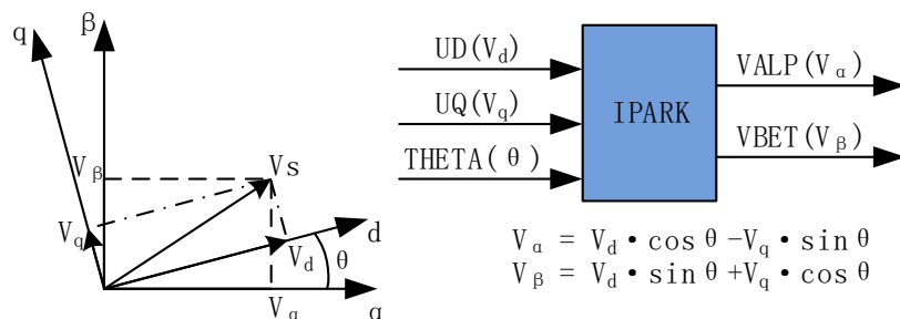
图 13-2 Park 逆变换
