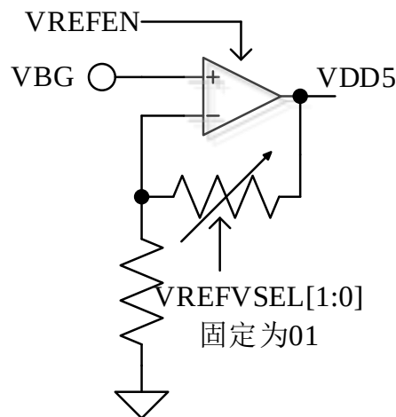
图 25-1 VREF 参考电压选择
