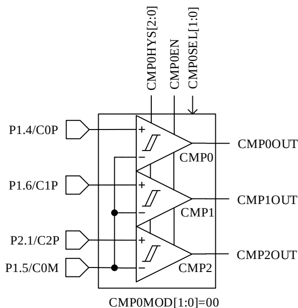
图 28-8 无内置电阻三比较器模式
