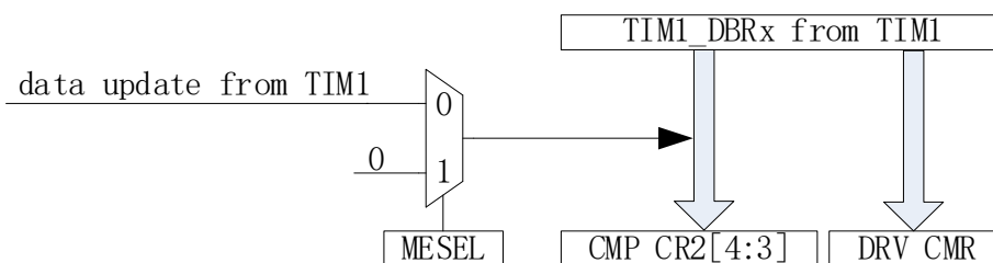
图 18-5 Timer1 自动控制 DRV_CMR 和 CMP_CR2[4:3]
