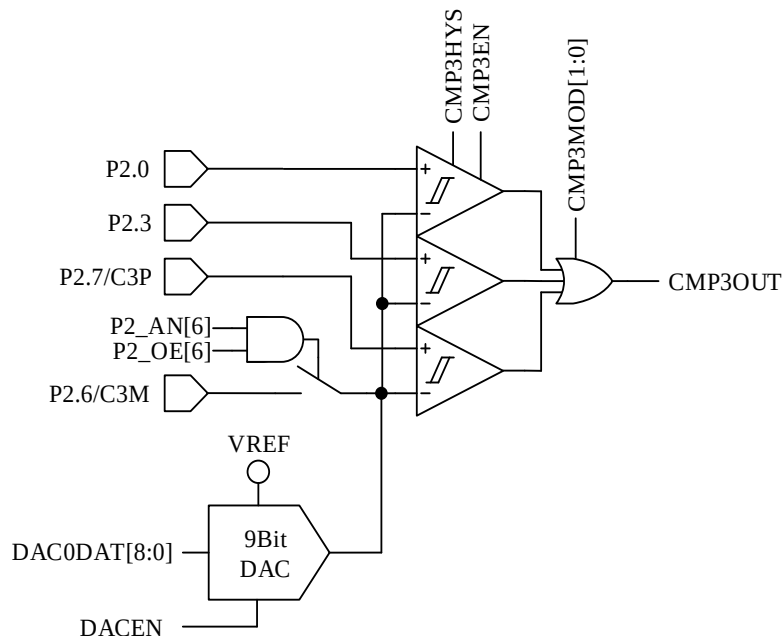
图 28-1 CMP3 的输入输出相关信号
