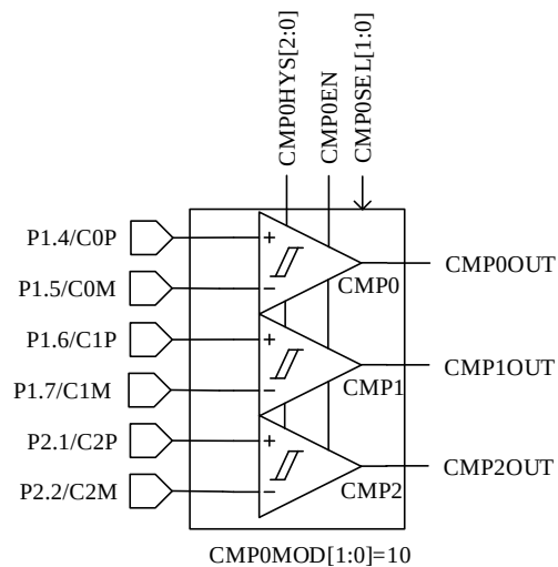
图 28-11 择差分三比较器模式
