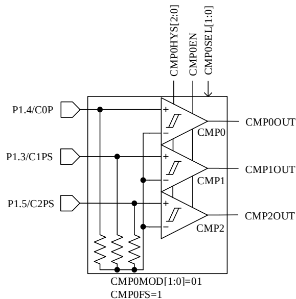
图 28-10 有内置电阻 3 比较器模式，端口功能转移
