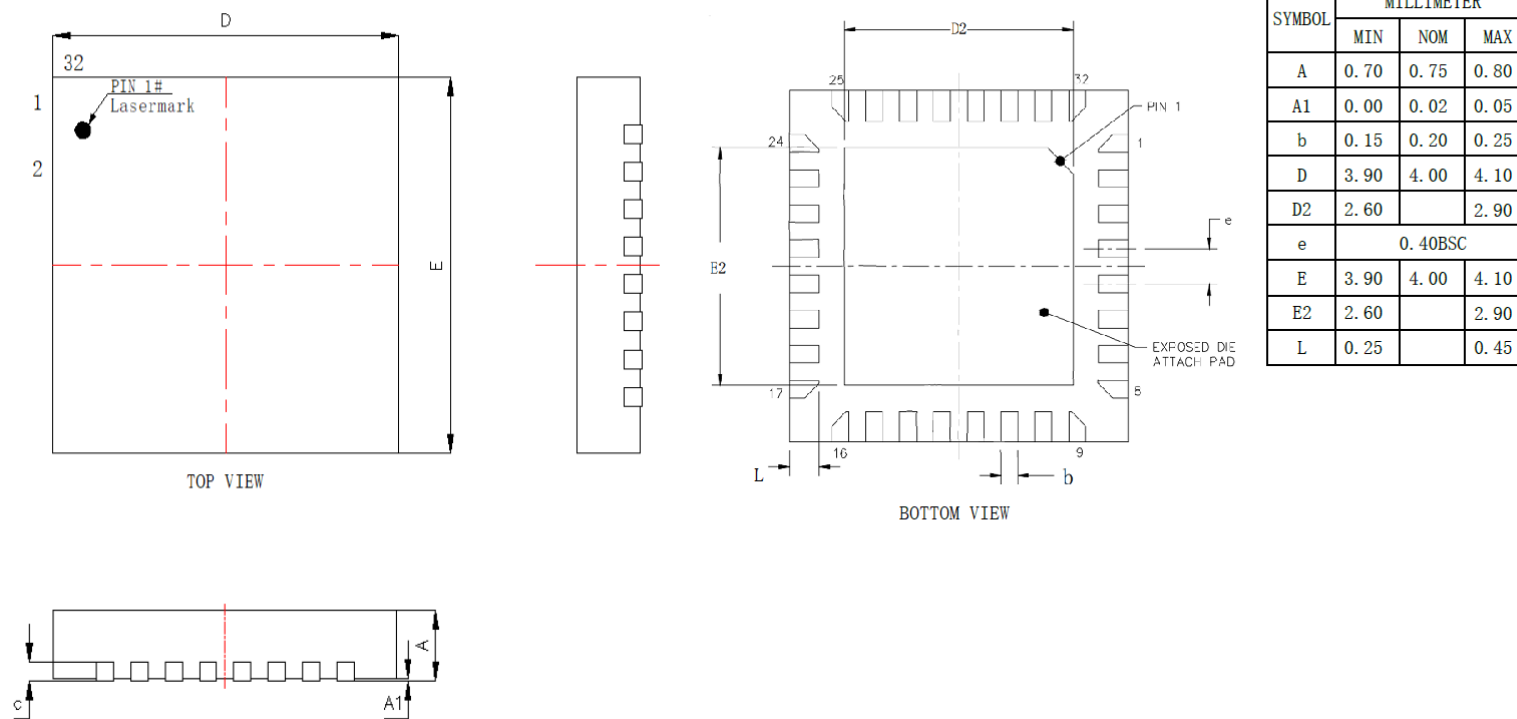
图 3-1 QFN32_4X4 封装尺寸图
