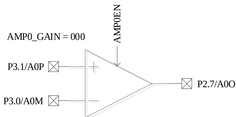
图 27-2 母线电流运放 AMP0
