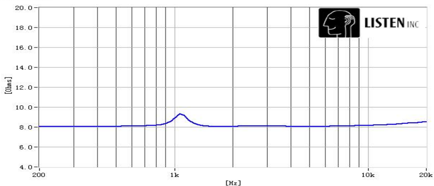
阻抗曲线
