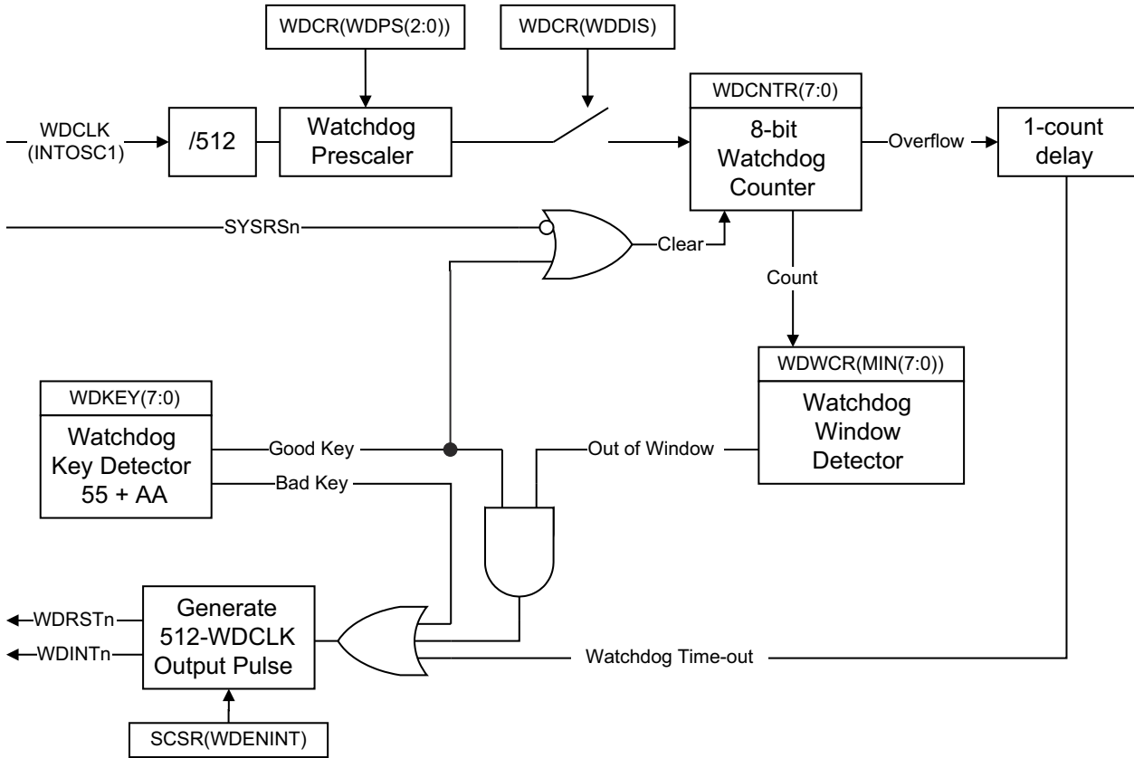
图 7-5. 窗口看门狗
