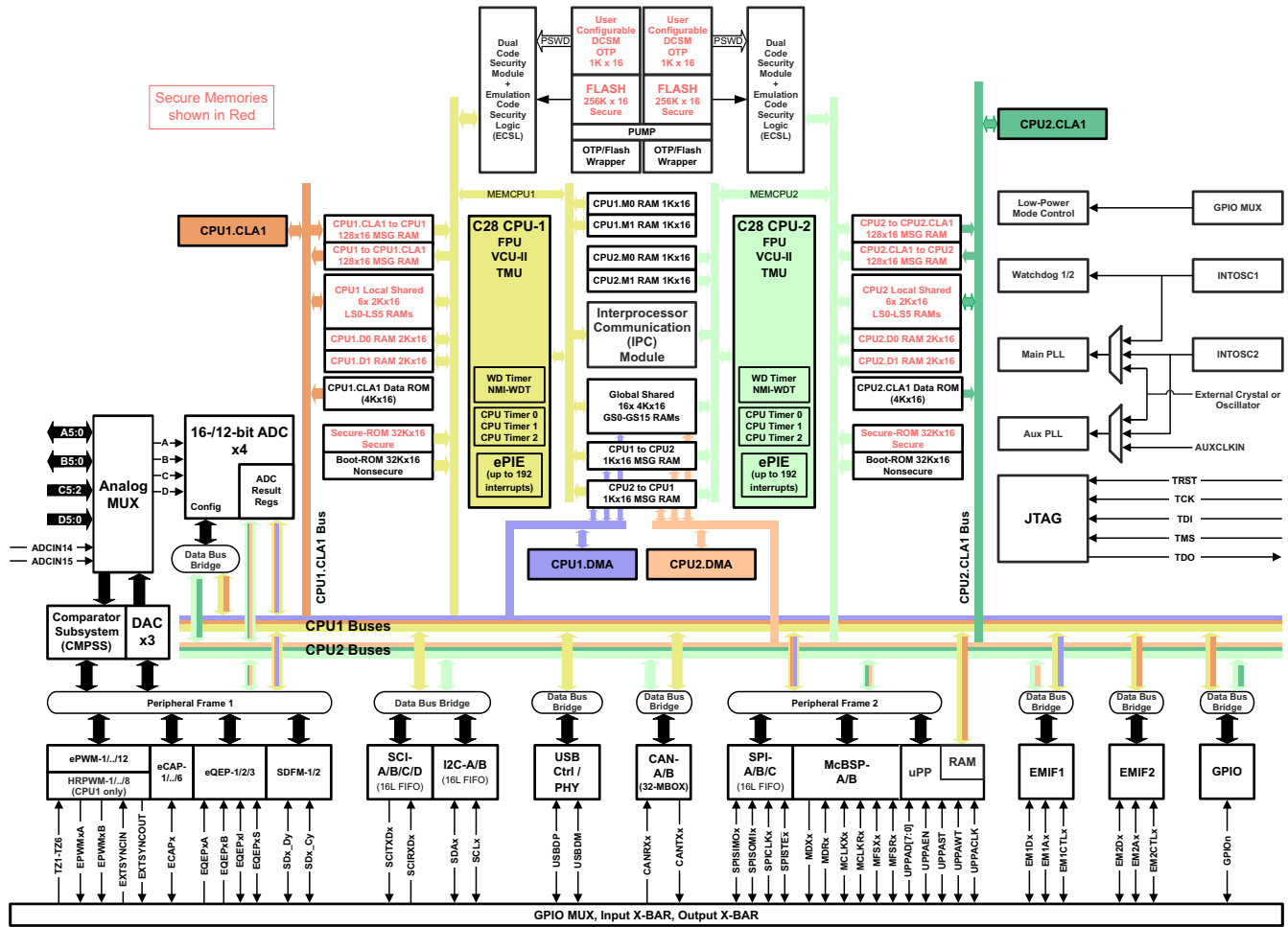
图 3-1. 功能方框图
