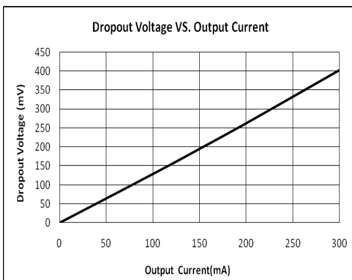
(8) 压差与输出电流 (QN73XXA50)
