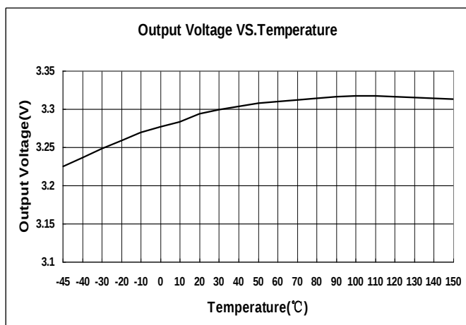
(9) 输出电压与温度 (QN73XXA33PG)
