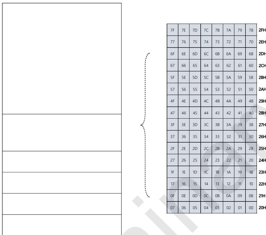
SRAM 结构图
