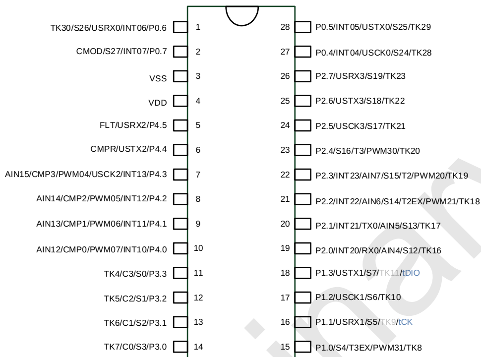
SC95F8763 管脚配置图 适用于 SOP28 及 TSSOP28 封装
