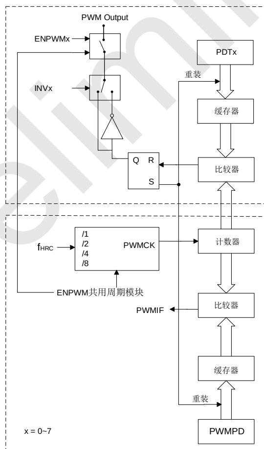
SC95F876X PWM 结构框图
