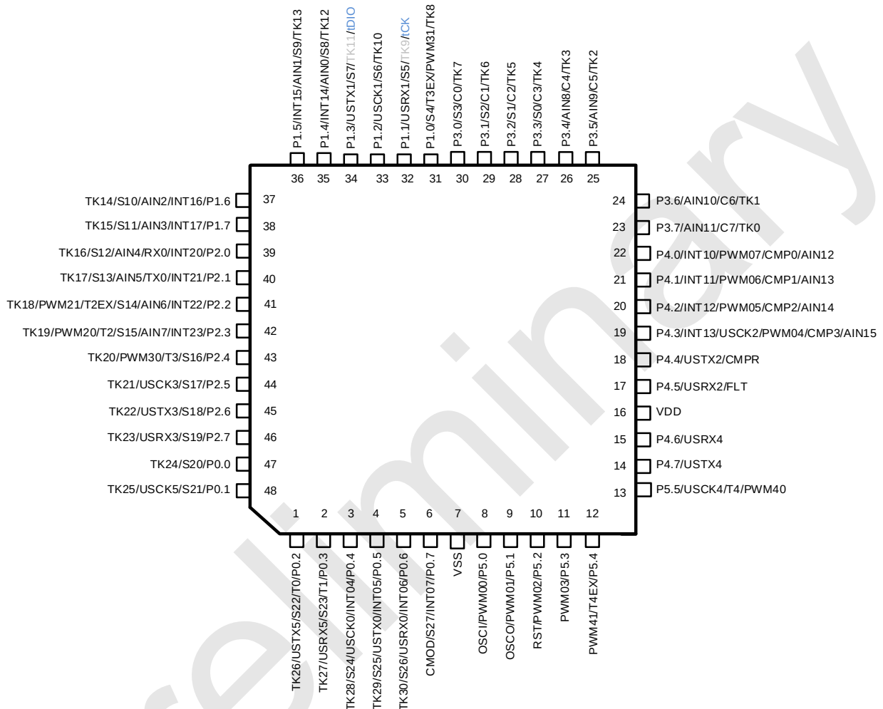
SC95F8767 管脚配置图 适用于 LQFP48、QFN48 封装
