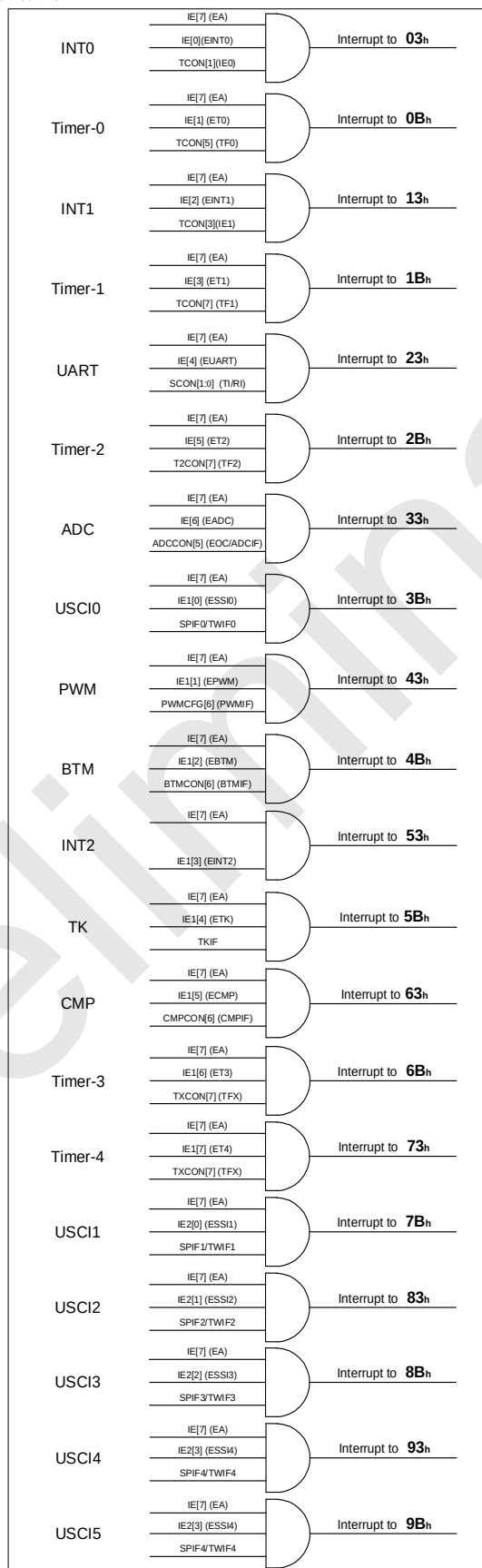
SC95F876X 中断结构和向量
