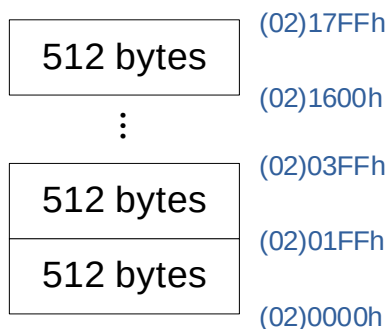
SC95F876X EEPROM Sector 分区示意
