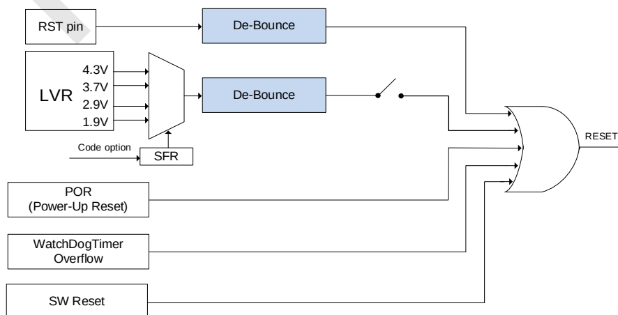
SC95F876X 复位电路图
