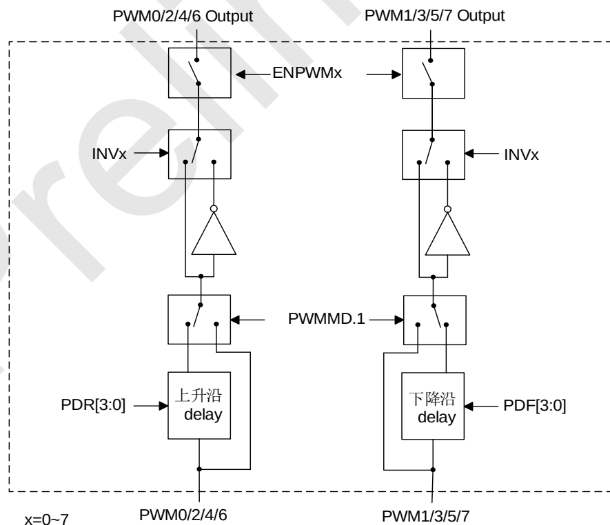
SC95F876X PWM 互补模式框图
