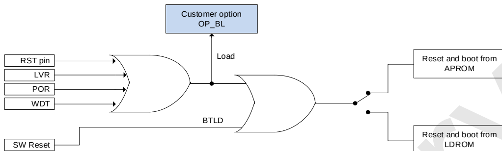
SC95F876X 复位后启动区域切换示意图
