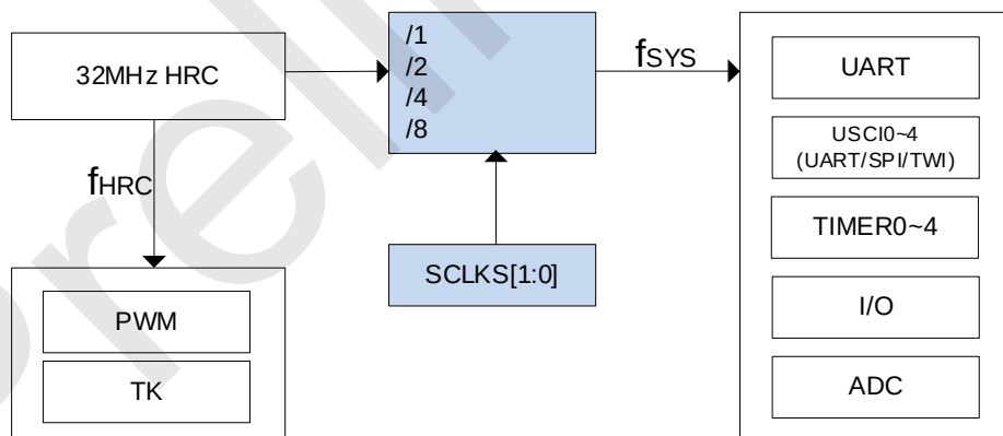
SC95F876X 内部时钟关系
