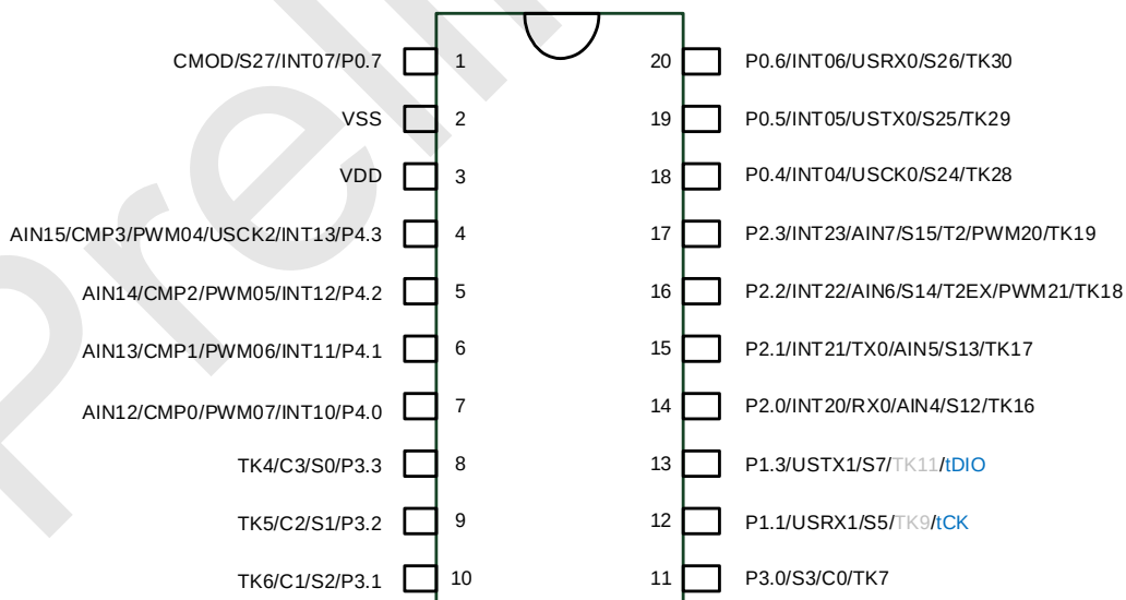
SC95F8762 管脚配置图 适用于 SOP20 及 TSSOP20 封装
