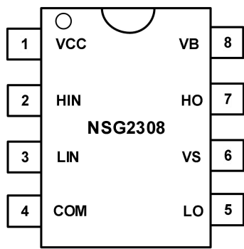
图 7-1 8-脚 SOP8 顶视图
