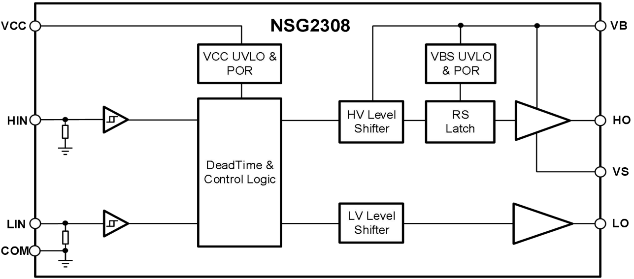
图 10-1 NSG2308 的功能框图
