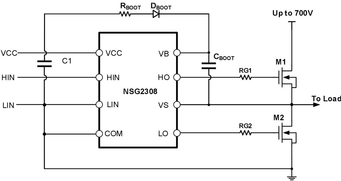
图 10-2 NSG2308 典型应用电路图
