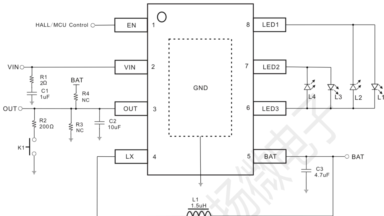
Fig1.LY6394E 典型应用电路
