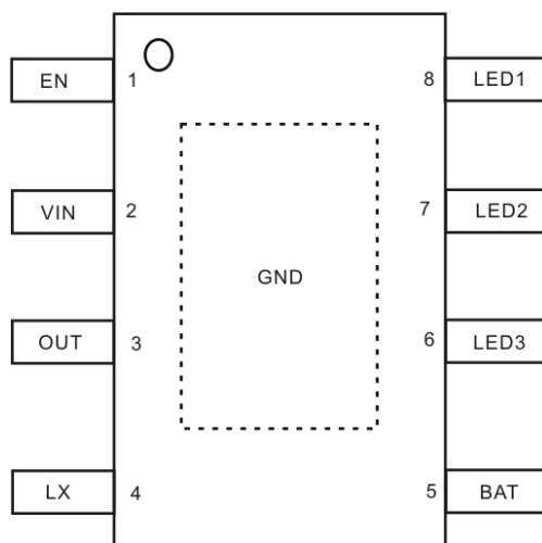
Fig4.管脚示意图
