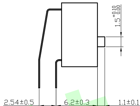
高推柄 High handle
