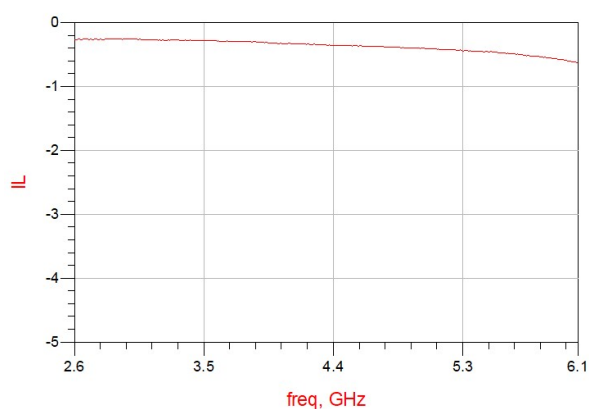
Figure 10. MHC4350L03 IL
