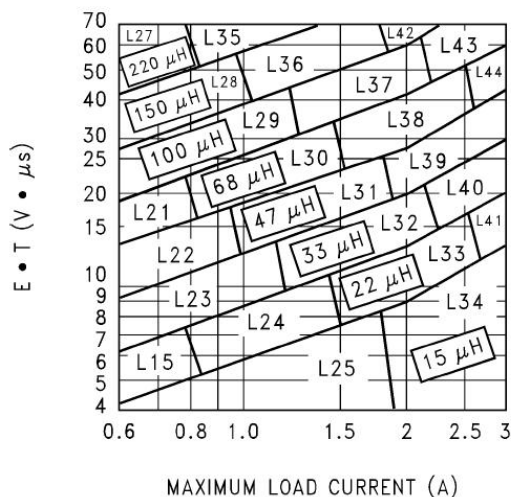
LM2596HV-ADJ
